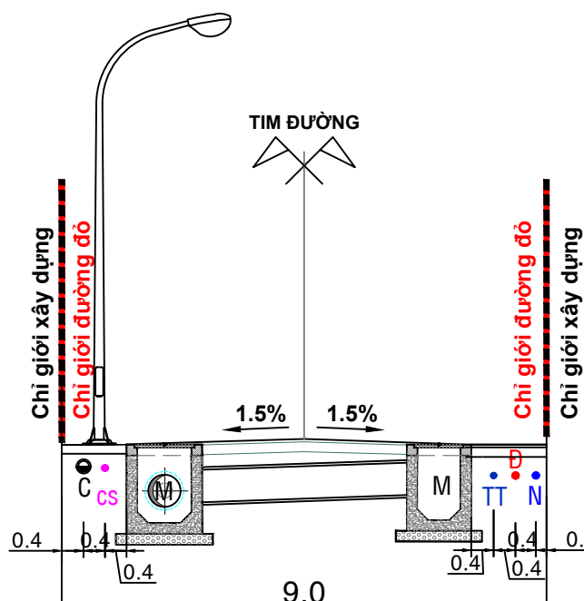
MẶT CẮT 1-1
