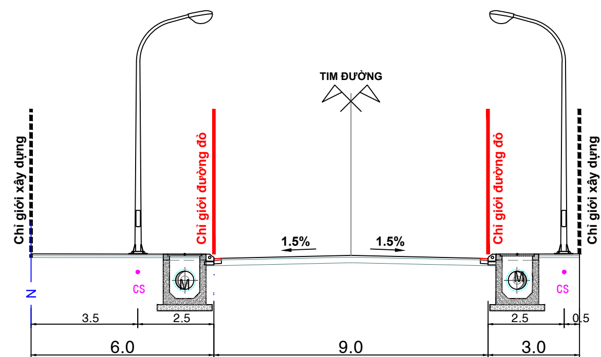
MẶT CẮT 2-2
