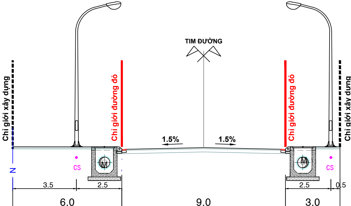
MẶT CẮT 2-2
