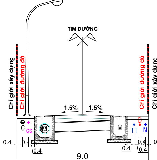
MẶT CẮT 1-1
